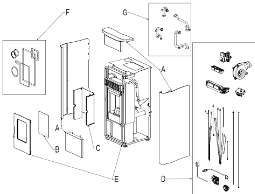
Fig. 1 - Esploso
