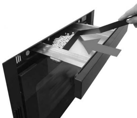
Fig. 35 - Pousser les granulés avec une petite pelle
