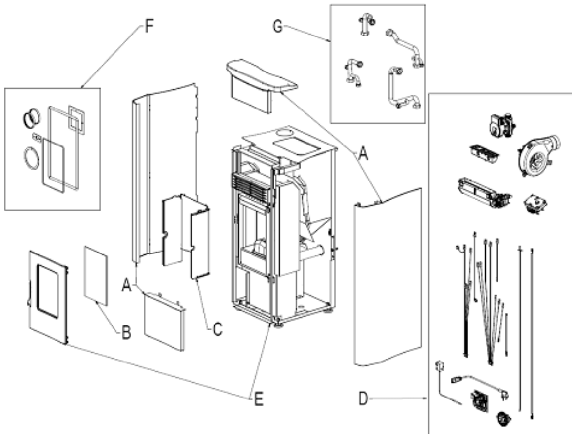
Fig. 1 - Dessin éclaté
