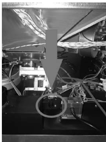
Fig. 42 - Réarmement manuel: il se trouve derrière le réservoir, près de la prise d'alimentation
