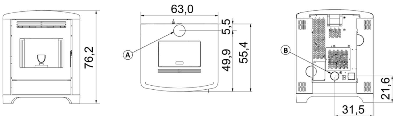
Fig. 12 - Dimensioni generali: MAGRITTE 6
