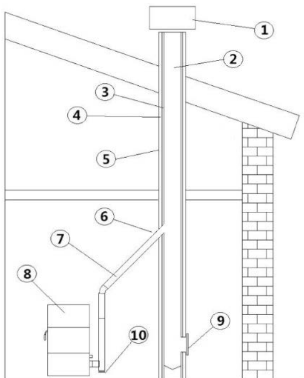
Fig. 2 - Componenti camino
