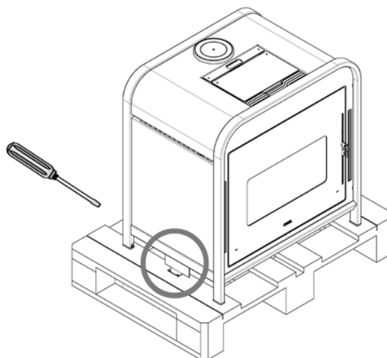
Fig. 1 - Rimozione viti + staffe
