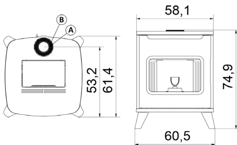
Fig. 13 - Dimensioni generali: HUBLLOT 6 UP
