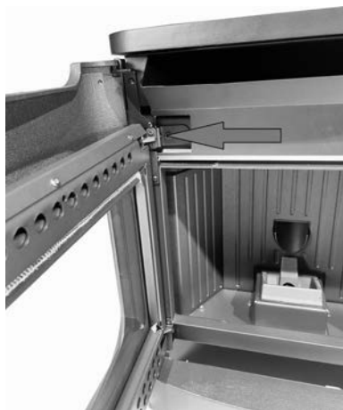
Fig. 17 - Regolazione porta
