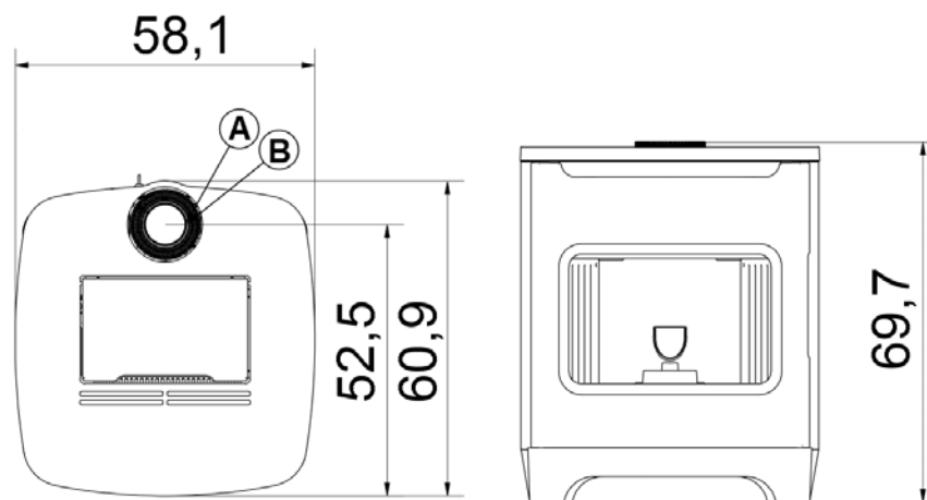
Fig. 14 - Dimensioni generali: FLOS 6
