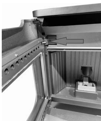
Fig. 19 - Regulación de la puerta
