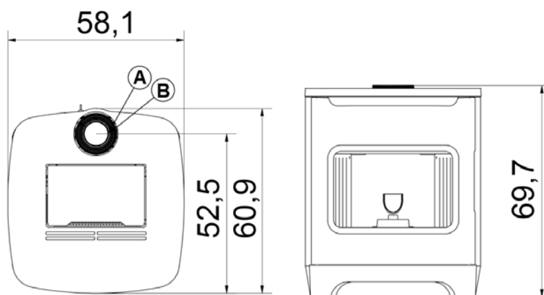
Fig. 16 - Dimensiones generales: FLOS 6
