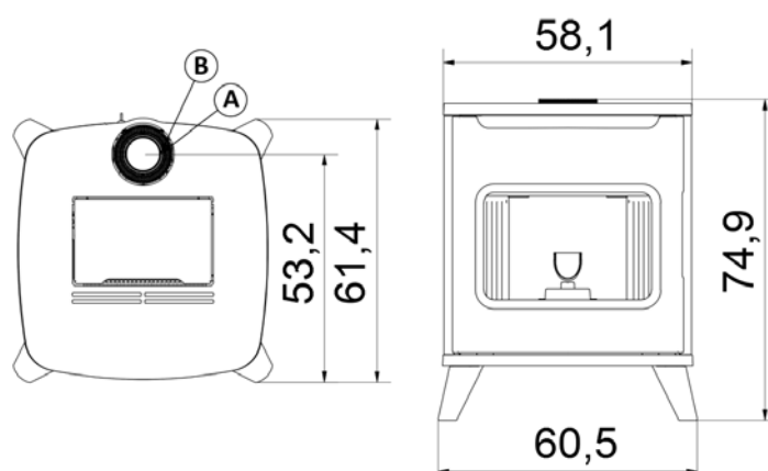
Fig. 15 - Dimensiones generales: HUBLLOT 6 UP
