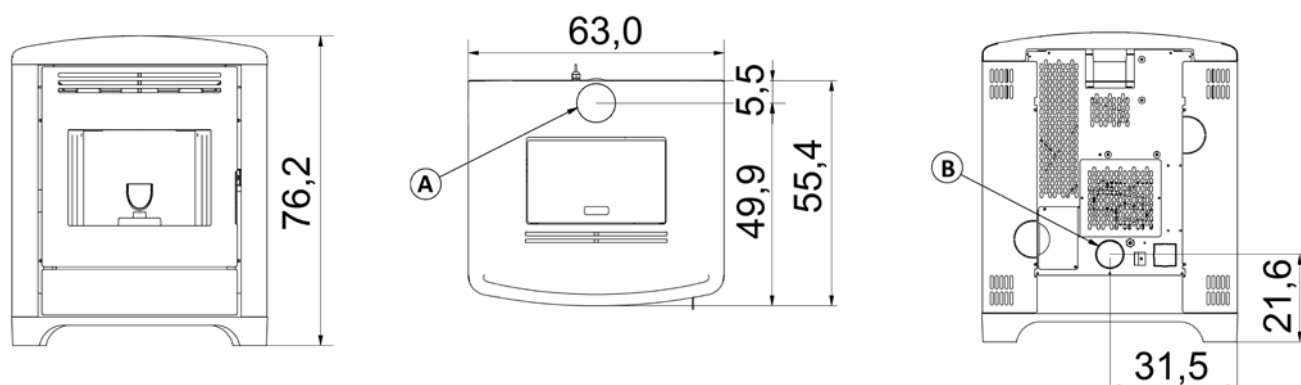
Fig. 14 - Dimensiones generales: MAGRITTE 6
