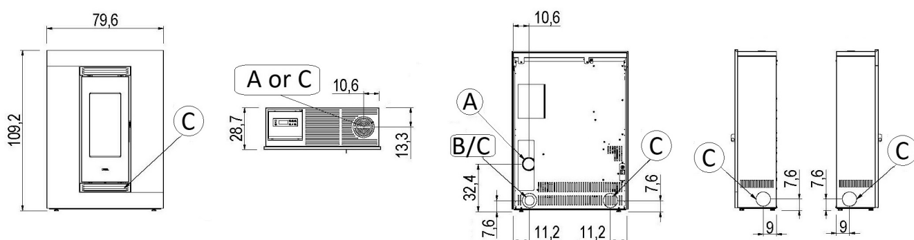
Fig. 12 - Dimensioni generali: Luce Plus 9
