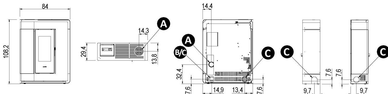
Fig. 14 - Dimensioni generali: Arco 7/9
