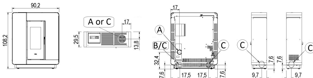
Fig. 13 - Dimensioni generali: Elle Plus 9
