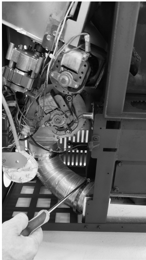
Fig. 26 - Svitare la Fascetta
