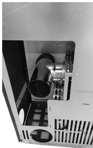
Fig. 38 - Collagare il tubo di scarico
