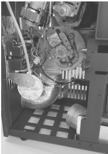
Fig. 29 - installare tubo flessibile
