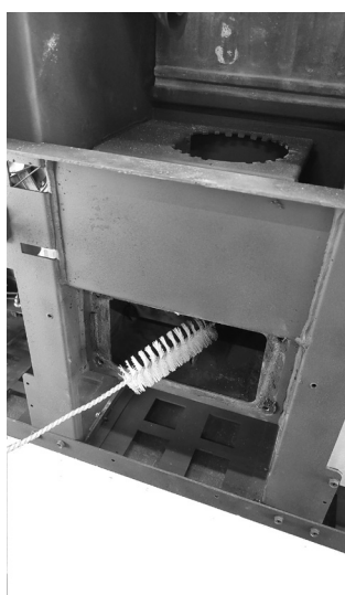
Fig. 51 - Pulire con scovolino
