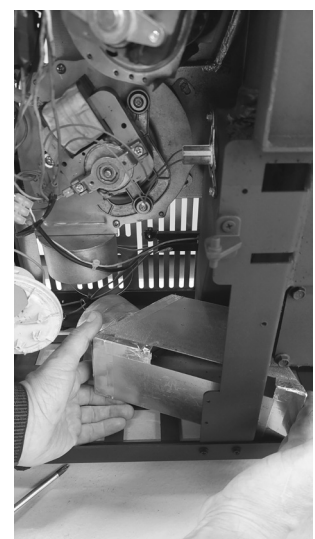
Fig. 31 - togliere la scatola
