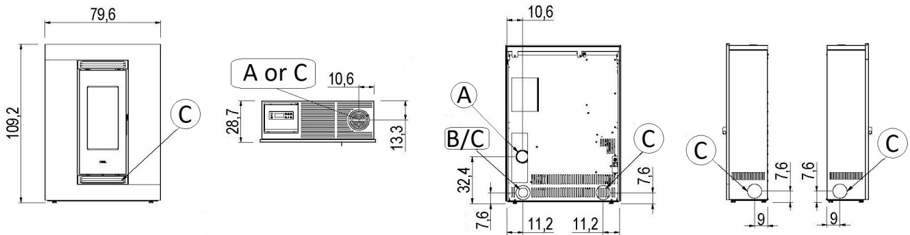
Fig. 21 - Dimensions générales: Luce Plus 9
