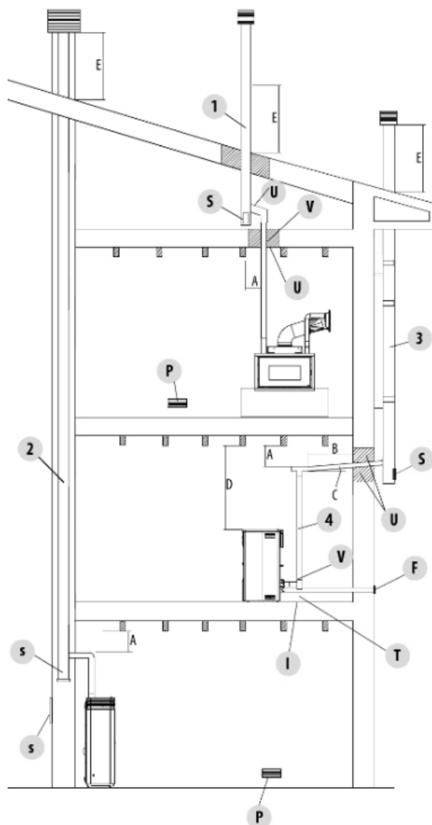
Fig. 11 - Conduit des fumées
