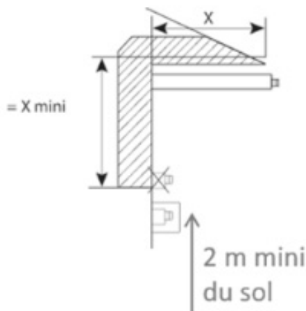
Fig. 14 - Rebord de toit
