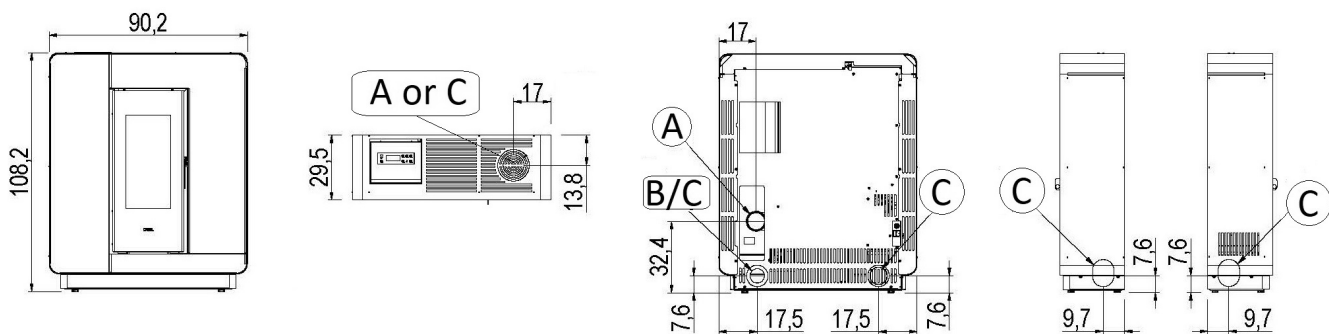
Fig. 22 - Dimensions générales: Elle Plus 9
