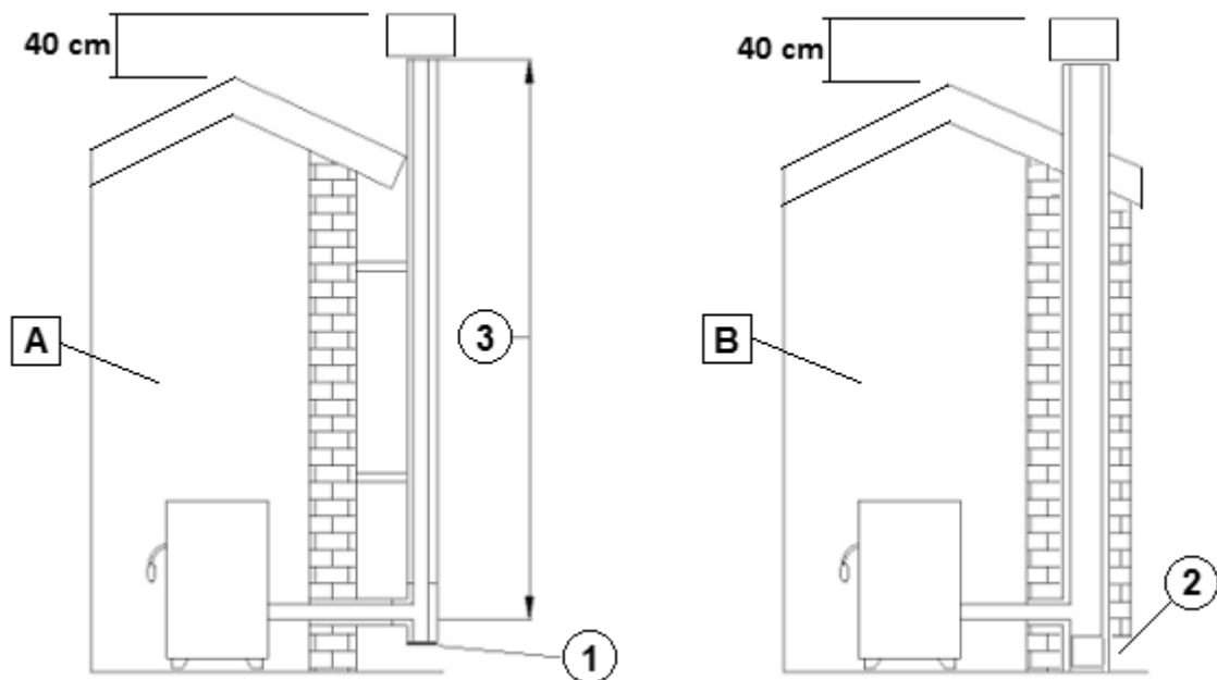
Fig. 3 - Conduit de fumées
