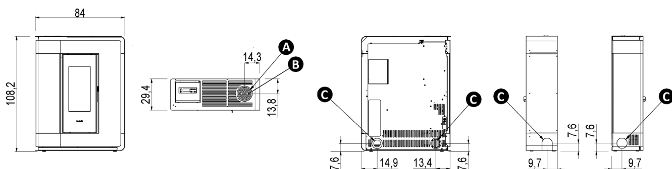
Fig. 24 - Dimensions générales: Arco 7/9 Bi-Flux
