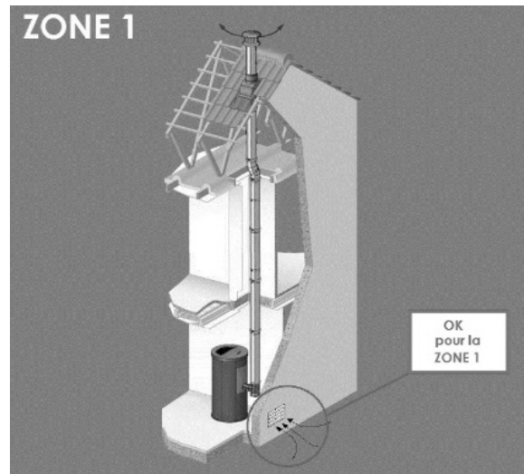
Fig. 15 - Installation possible pour tous les poêles (ZONE 1)
