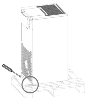
Fig. 1 - Retrait des étriers
