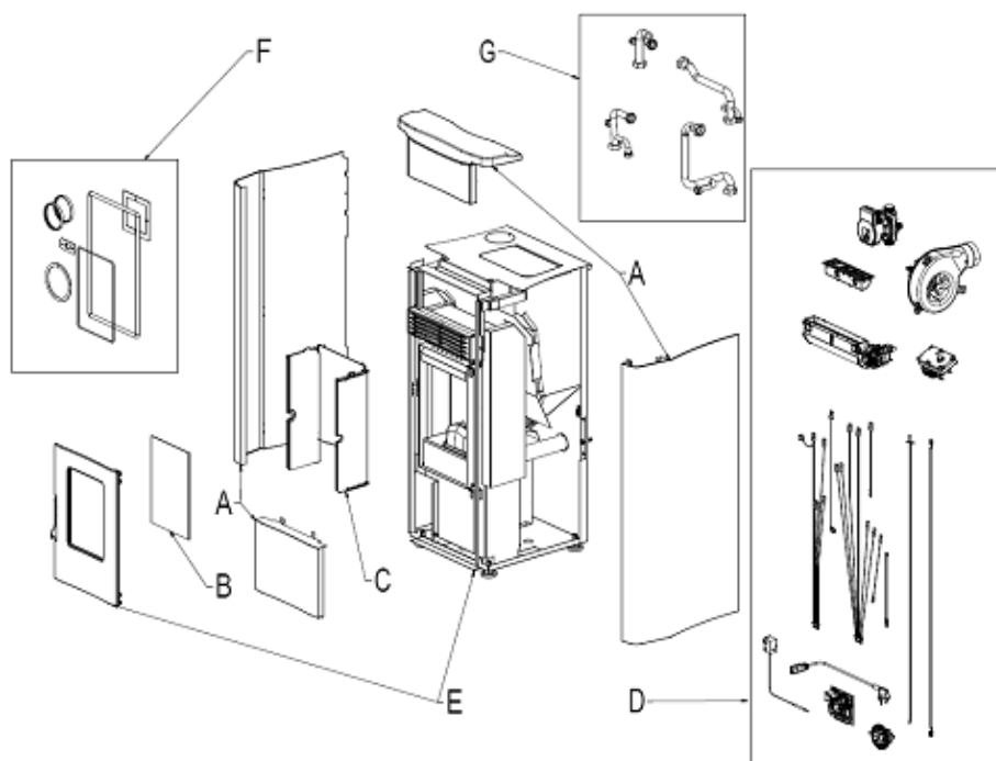
Fig. 1 - Explosionszeichnung
