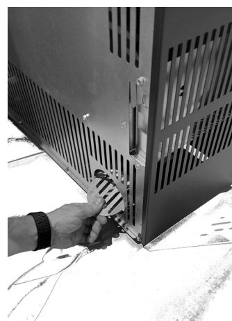
Fig. 31 - Paso del tubo
