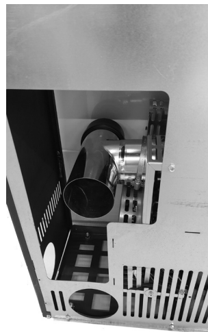
Fig. 41 - Conexión de la descarga de humos
