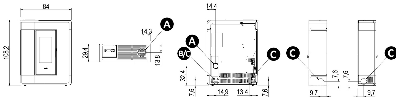
Fig. 17 - Dimensiones generales: Arco 7/9
