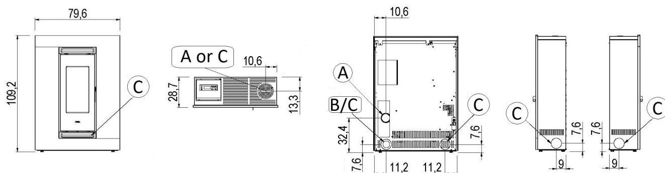
Fig. 15 - Dimensiones generales: Luce Plus 9
