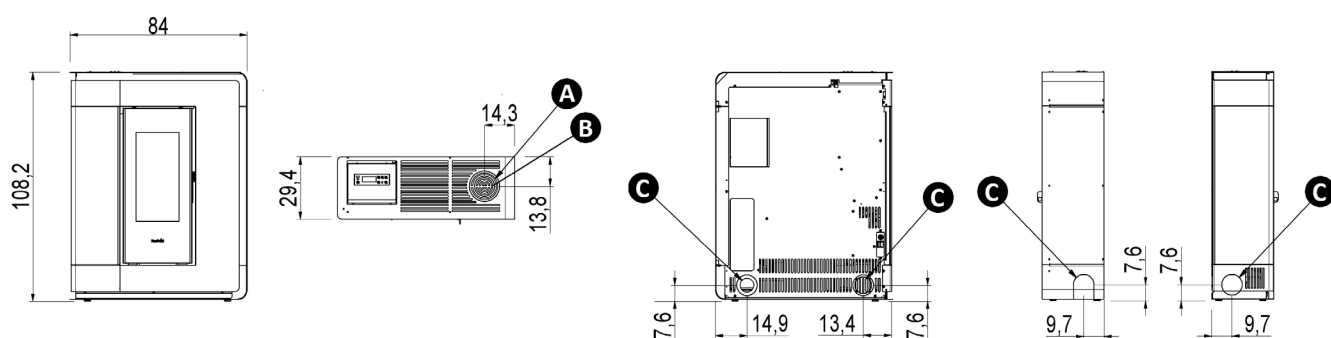
Fig. 18 - Dimensiones generales: Arco 7/9 Bi-Flux
