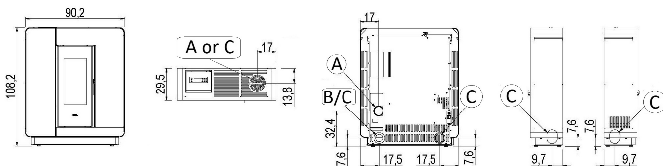
Fig. 16 - Dimensiones generales: Elle Plus 9
